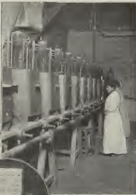
Serie de sopletes de gas oxhídrico encerrados en una envoltura de palastro, en la cual hay una ventanilla con un cristal por la que la obrera vigila el curso de la operación.
